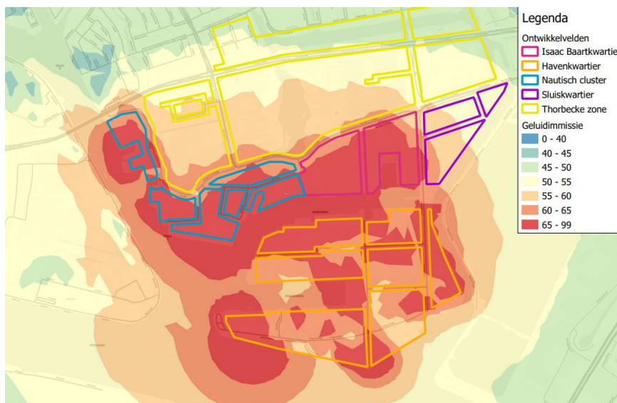
Figuur 2.4 Geluidbelasting (op 5 meter), met maximale invulling van het zonemodel in de deelgebieden Nautisch cluster, Isaac Baartkwartier en Havenkwartier.
