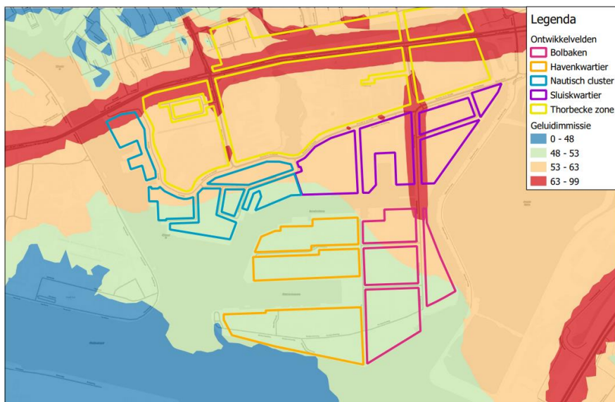
Figuur 3.4 Wegverkeerslawaai in de plansituatie (op 5 meter hoogte)
